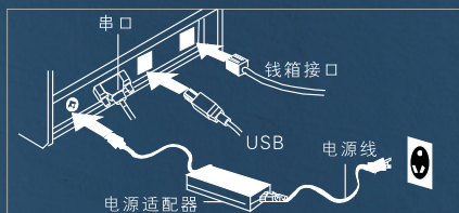
打印机连接示意图：
